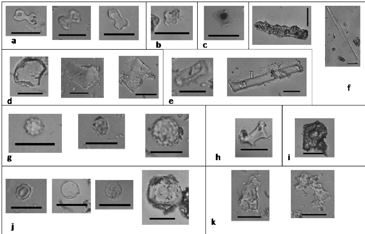
Figure 4: Microphotograph Phytoliths morphotypes: Poaceae: a) bilobates; b)cross; c) rondel; d) bulliform; e) trapeziform; f) elongate; Arecaceae: g) globular echinate; Chusquea: h) chusquea morphotype; Ciperaceae: i) ciperous morphotype; Eudicotiledoneae: j) globular ; Marantae: k)irregular faceted (magnification 40X). Bar=10µm
